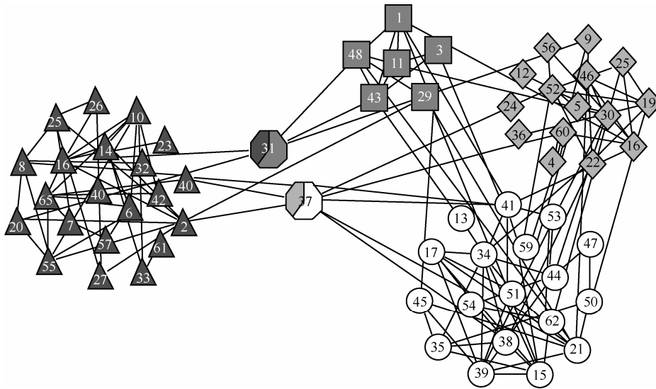
图 9 OMKLP 算法面对 Dolphins 所得到的社区结构
